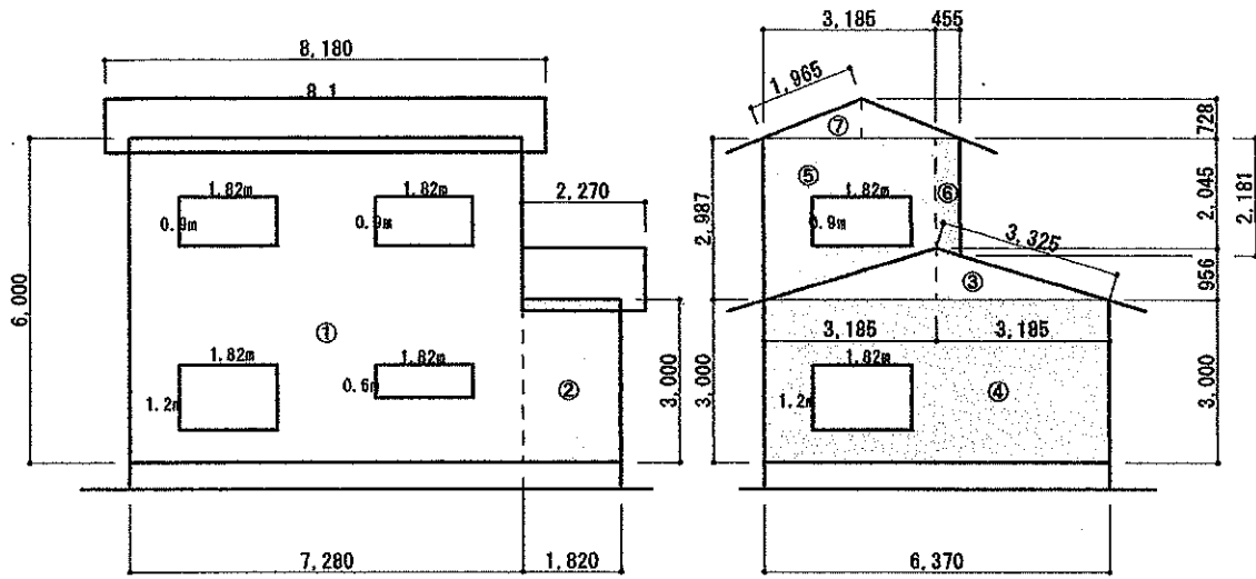
東立面图
